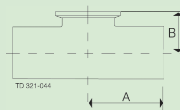
RACCORD EN T SOUDURE/SOUDURE/CLAMP COURT TRI-CLOVER CODE B7WWMS ASME BPE CODE DT-4.1.2-2
