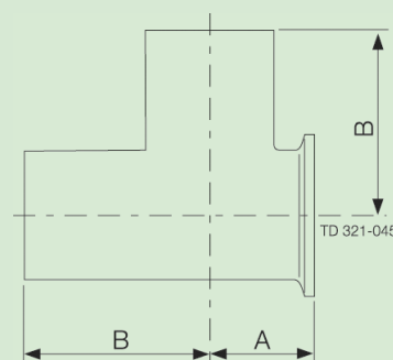
RACCORD EN T SOUDURE/CLAMP/SOUDURE "OUTLET RUN" TEE TRI-CLOVER CODE B7WMSW ASME BPE CODE DT-4.1.2-3
