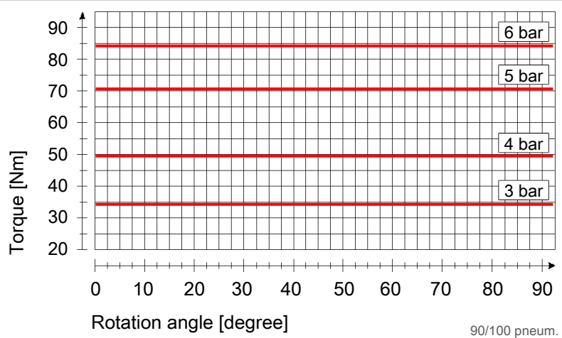
90/ 100 air / air
