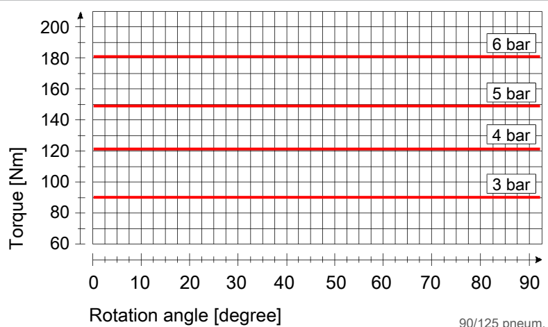
90/ 125 air / air
