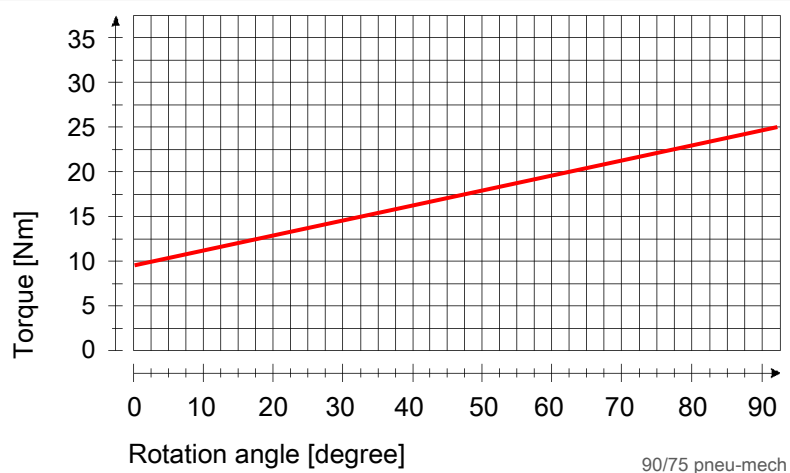
90/ 75 air / spring
