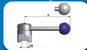
Handbediening SV04 traploos instelbaar
