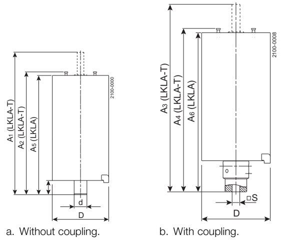
Fig. 2. Dimensions - actuator.
