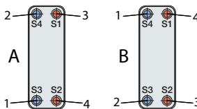
Figuur 5. Enkel circuit: A verdamper; B condensor.
