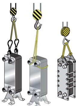
Figuur 2. Voorbeelden van hijsen.
