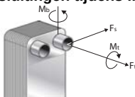
Figuur 3. Belasting op de aansluitingen.
