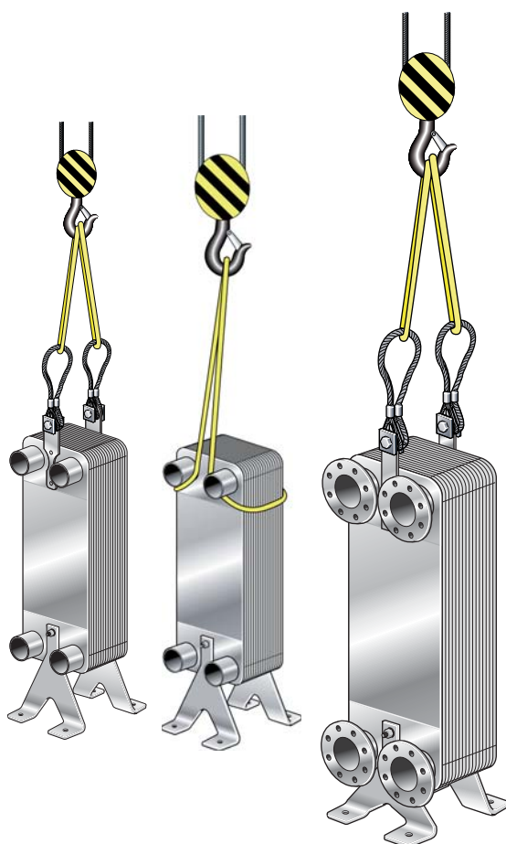
Figuur 2. Voorbeelden van hijsen.
