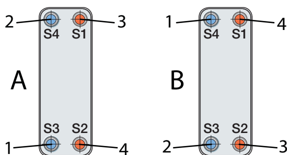
Figuur 5. Enkel circuit: A verdamper; B condensor.
