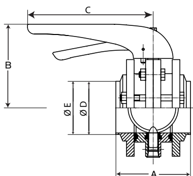
SVS1F Scheibenventil mit Handhebel
