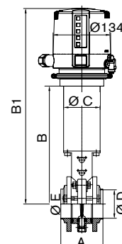
SVS1F Scheibenventil mit Standard-Drehantrieb oder Drehantrieb und Control Unit
