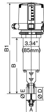
SV1 Scheibenventil mit Drehantrieb und Control Unit
