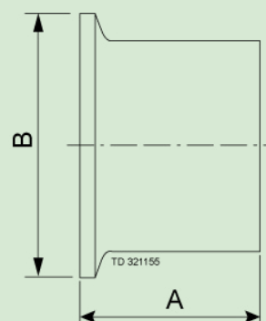
LASFERRULE MEDIUM / CLAMPFERRULE MEDIUM TRI-CLOVER CODE L14AM ASME BPE CODE DT-4.1.4-1 (VOORHEEN DT-22B)
