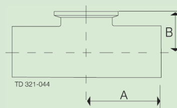
T-STÜCK SCHWEISS/SCHWEISS/CLAMP KURZ TRI-CLOVER CODE B7WWMS ASME BPE CODE DT-4.1.2-2
