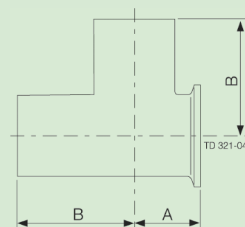
T-STÜCK SCHWEISS/SCHWEISS/CLAMP KURZOUTLET RUN TEE TRI-CLOVER CODE B7WMSW ASME BPE
